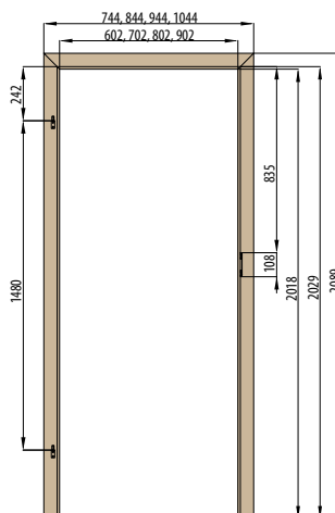
OŚCIEŻNICA REGULOWANA DO DRZWI SZKŁANYCH
