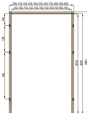
Kątownik standardowy do ościeżnicy regulowanej
