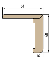
Kątownik z przedłużonym piórem do ościeżnicy regulowanej
